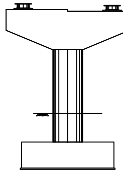
배면
